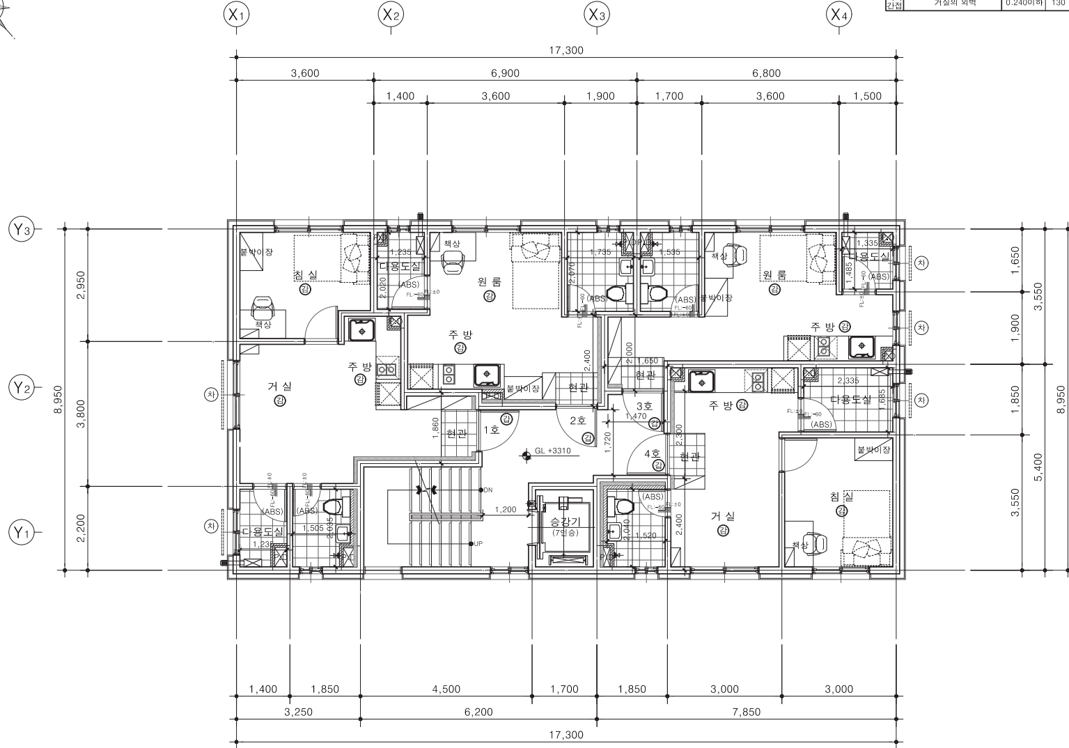
1 지상 2층 평면도 축척 - A3 : 1/100
