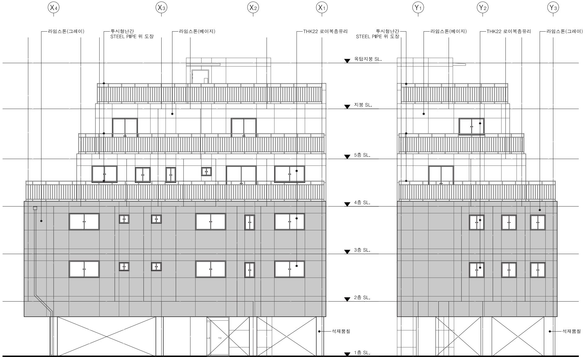
1 배 면 도 축척 - A3 : 1/100
