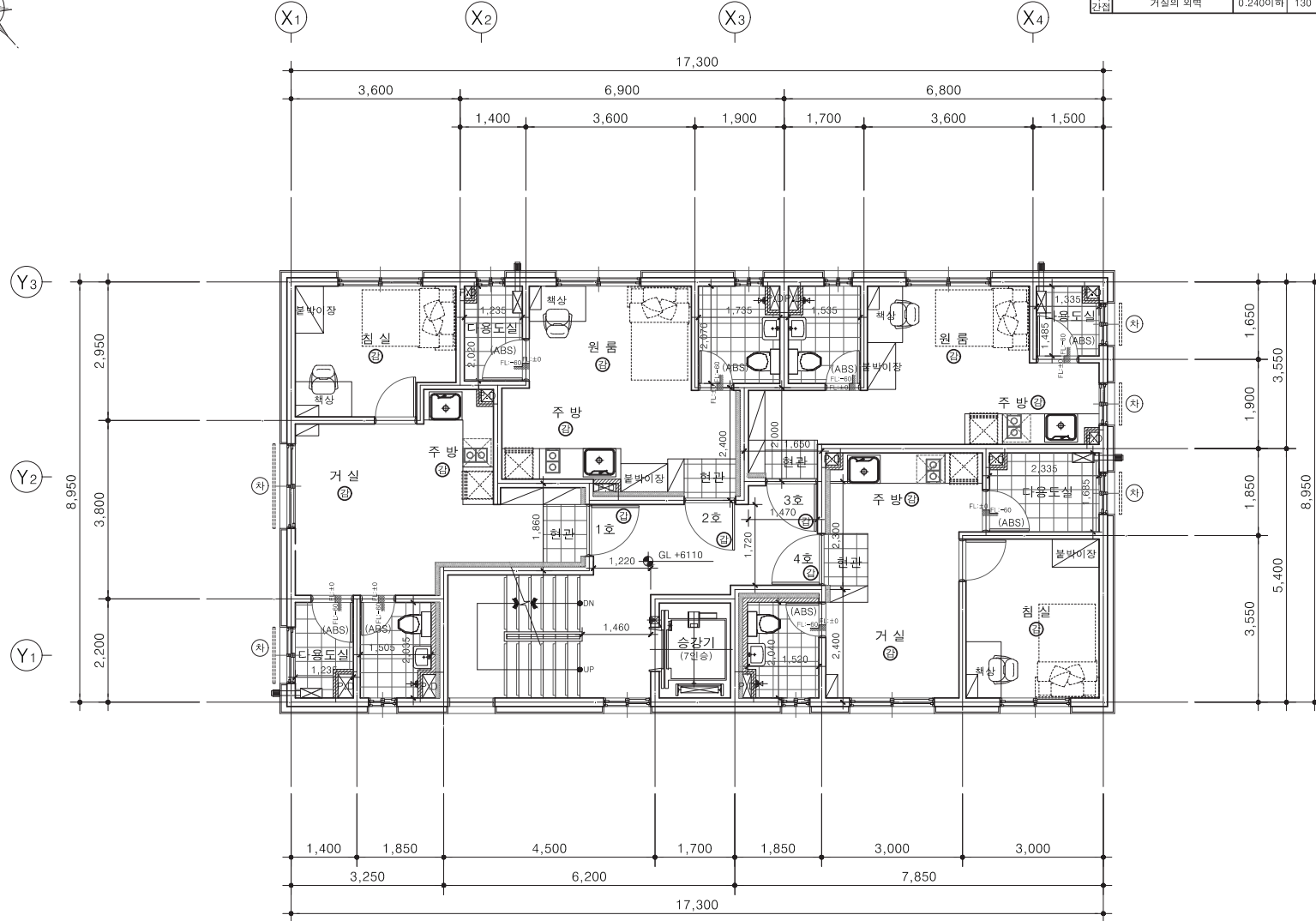
1 지상 3층 평면도 축척 - A3 : 1/100
