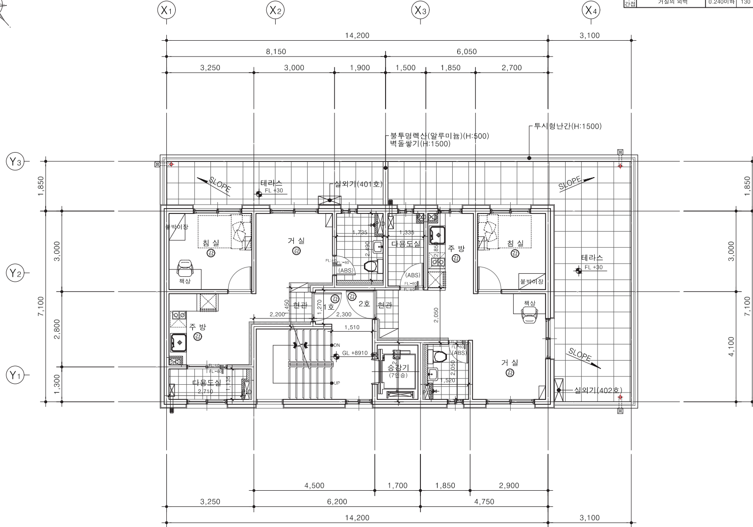
1 지상 4층 평면도 축척 - A3 : 1/100
