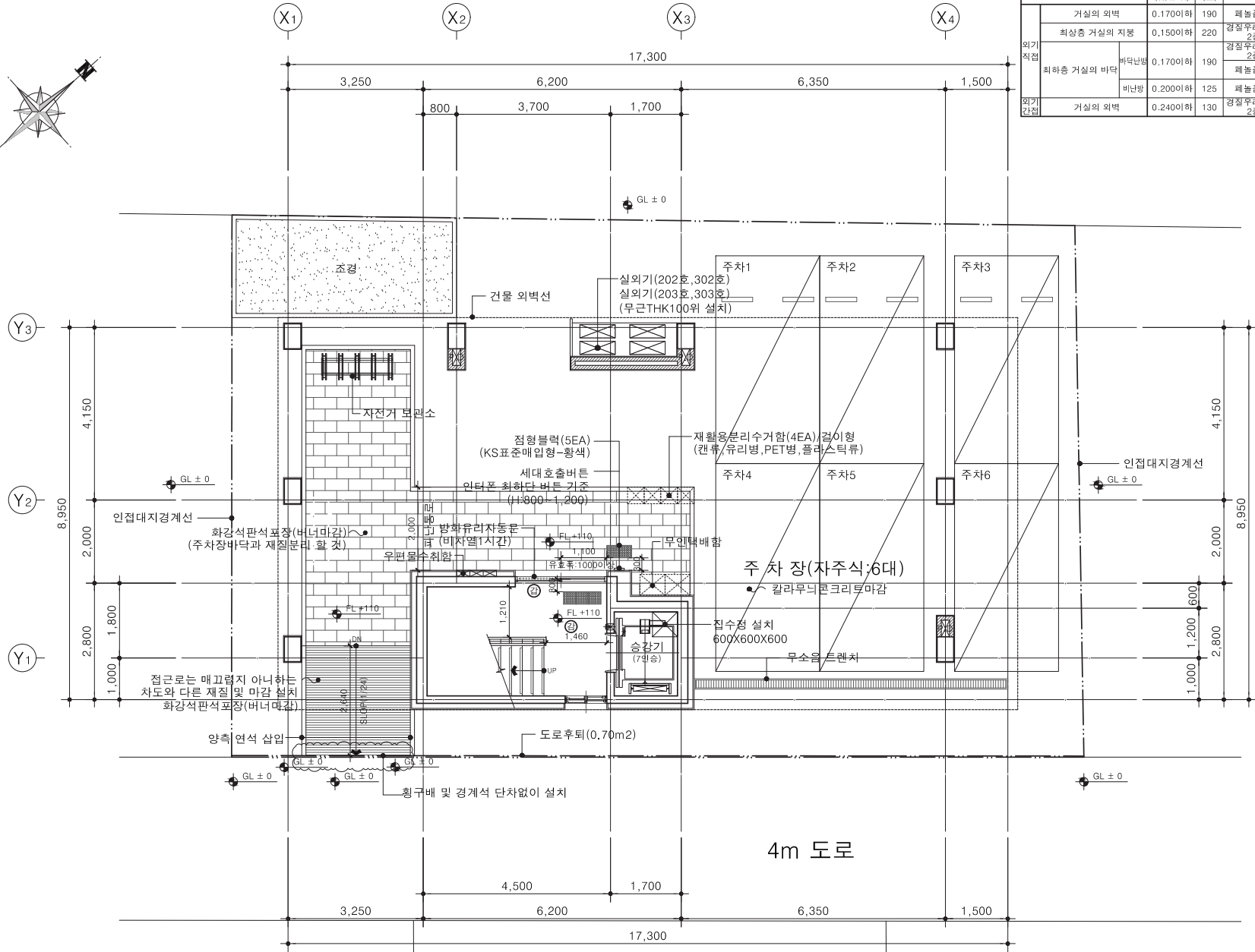
1 지상 1층 평면도 축척 - A3 : 1/100
