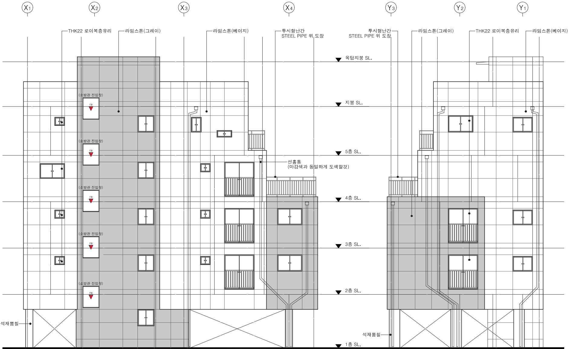
1 정 면 도 축척 - A3 : 1/100
