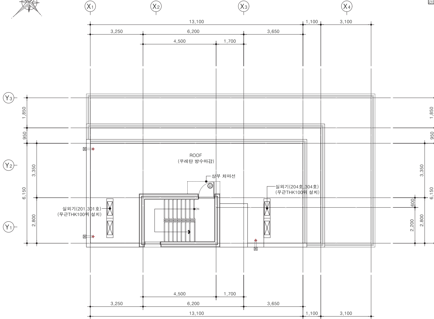
1 지붕 평면도 축척 - A3 : 1/100
