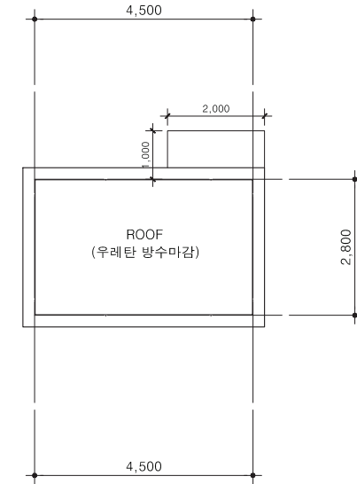
2 옥탑지붕 평면도 축척 - A3 : 1/100
