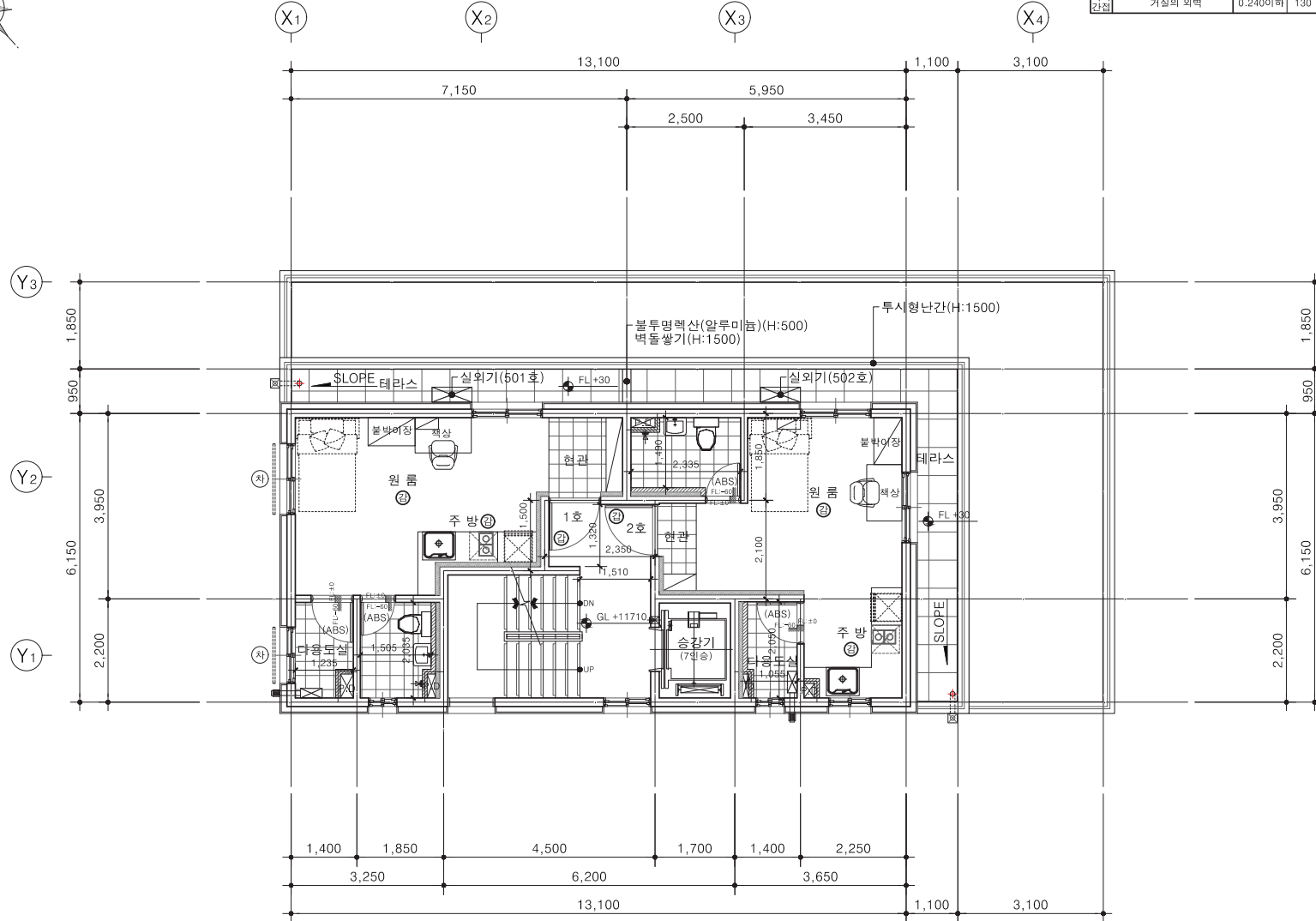
1 지상 5층 평면도 축척 - A3 : 1/100
